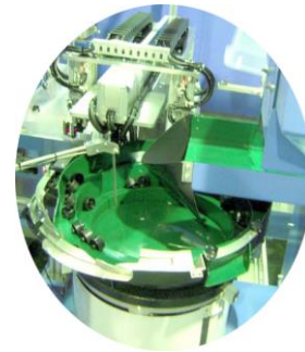
フット(足)の供給(方向性あり)
